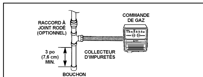
FIGURE 12 TUYAUTERIE DE GAZ AVEC RACCORD FLEXIBLE
