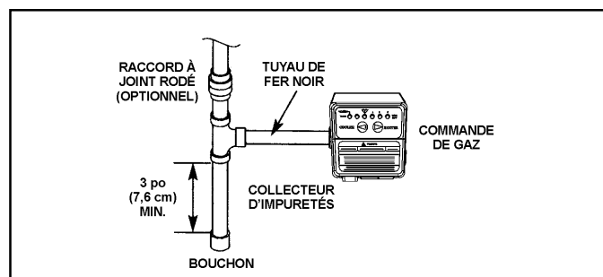
FIGURE 13 TUYAUTERIE DE GAZ AVEC TUYAU DE FER NOIR MENANT À LA COMMANDE DE GAZ
